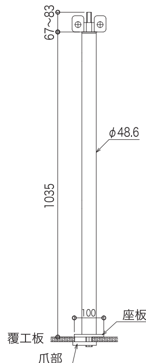
●ガードポスト(覆工板用)
