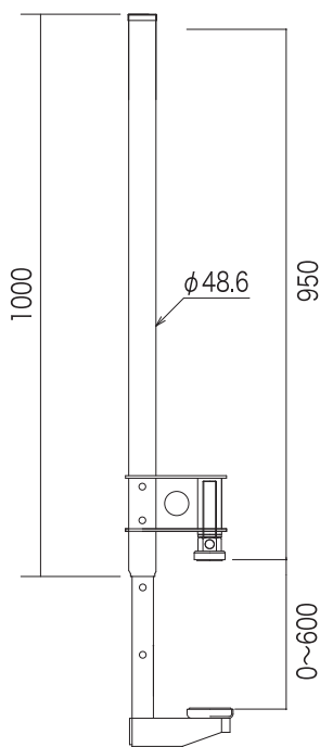
●スタンションNRE型
