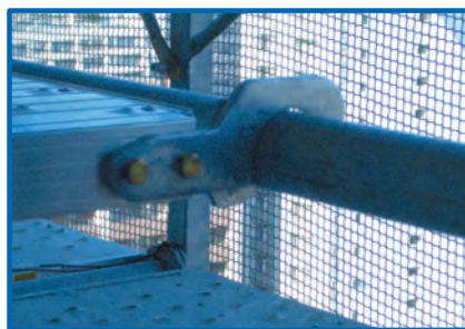
●フックは φ48.6・φ42.7
