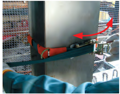
③バックルを作動させて締めこむ
